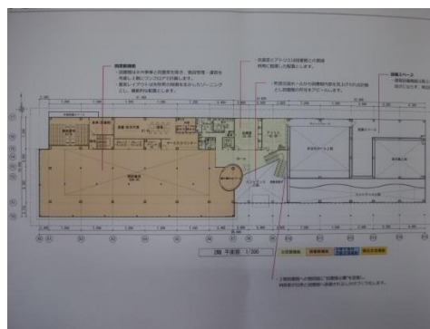
二階平面図
