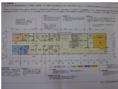
一階平面図
