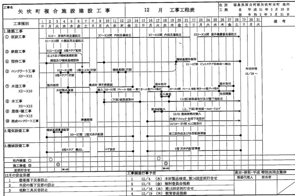
月間工程表
