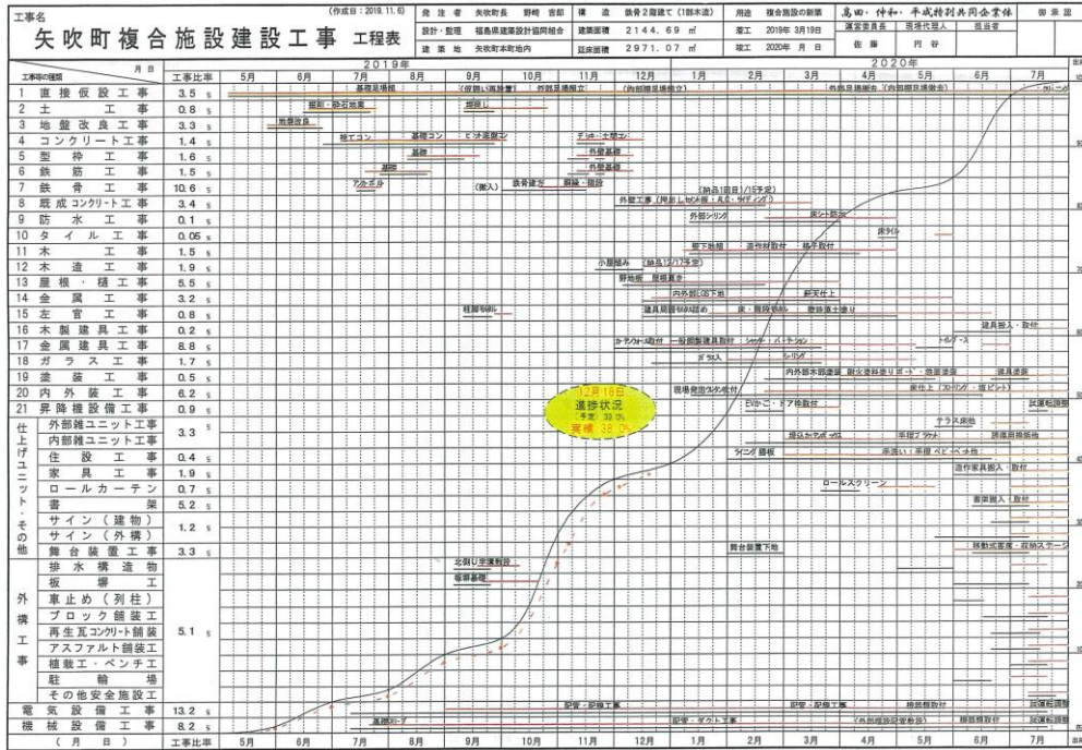
全体工程表
