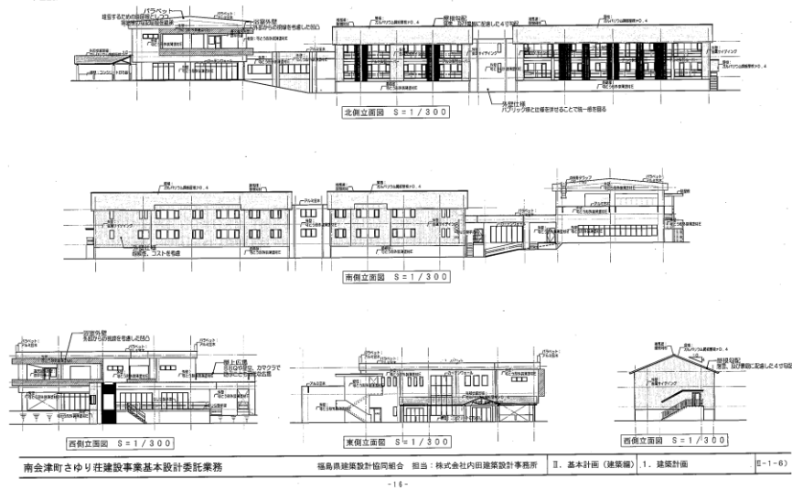
立面図（敷地に高低差有り）
